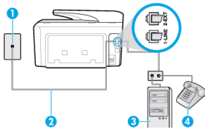
图 5-16 打印机的后视图
