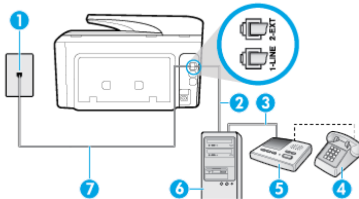
图 5-13 打印机的后视图
